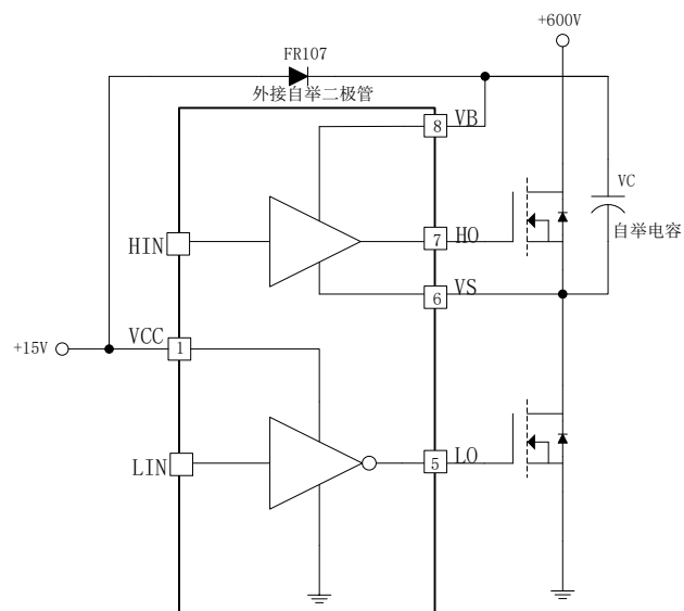
图 8-3. EG2101 自举电路结构
