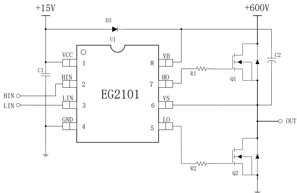
图 6-1. EG2101 典型应用电路图
