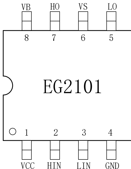
图 4-1. EG2101 管脚定义
