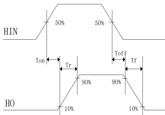
7-2. 高端输出 H0 开关时间波形图
