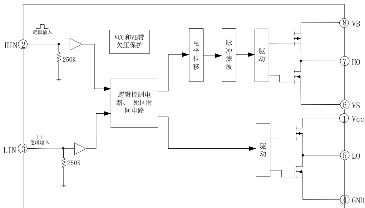
图 5-1. EG2101 内部电路图
